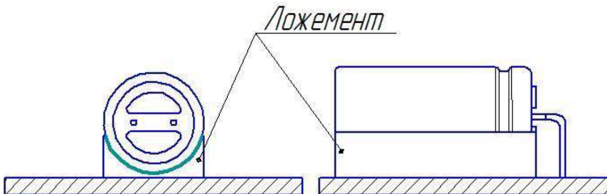
Рисунок Е.1 – Способ крепления конденсаторов в аппаратуре – за корпус приклеивкой клеем БФ-4 ГОСТ 12172 (или аналогичный) к ложементу и с закреплением выводов пайкой
